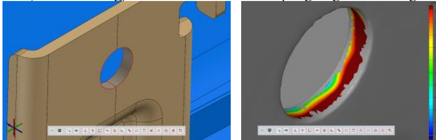
5. ábra: Hengeresség megjelenítése vizuálisan (szintérvéggel)
