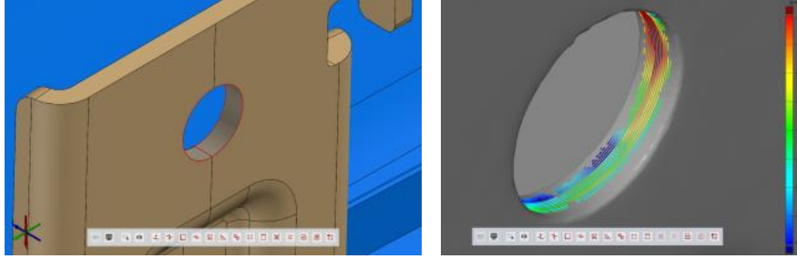
4. ábra: Körkörösség megjelenítése vizuálisan (szintérvéggel)
