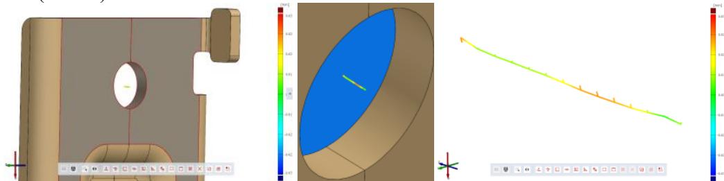
8. ábra: Merőlegesség megjelenítése vizuálisan (színtérképpel)
