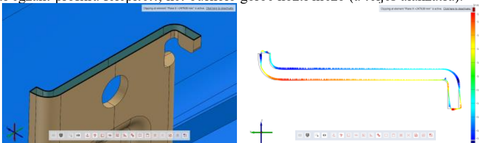
6. ábra: Kontúr (vonal) eltérés megjelenítése vizuálisan (szintérvéggel)
