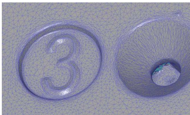
1. kép STL modell, azaz poligonizált pontfelhő képe
